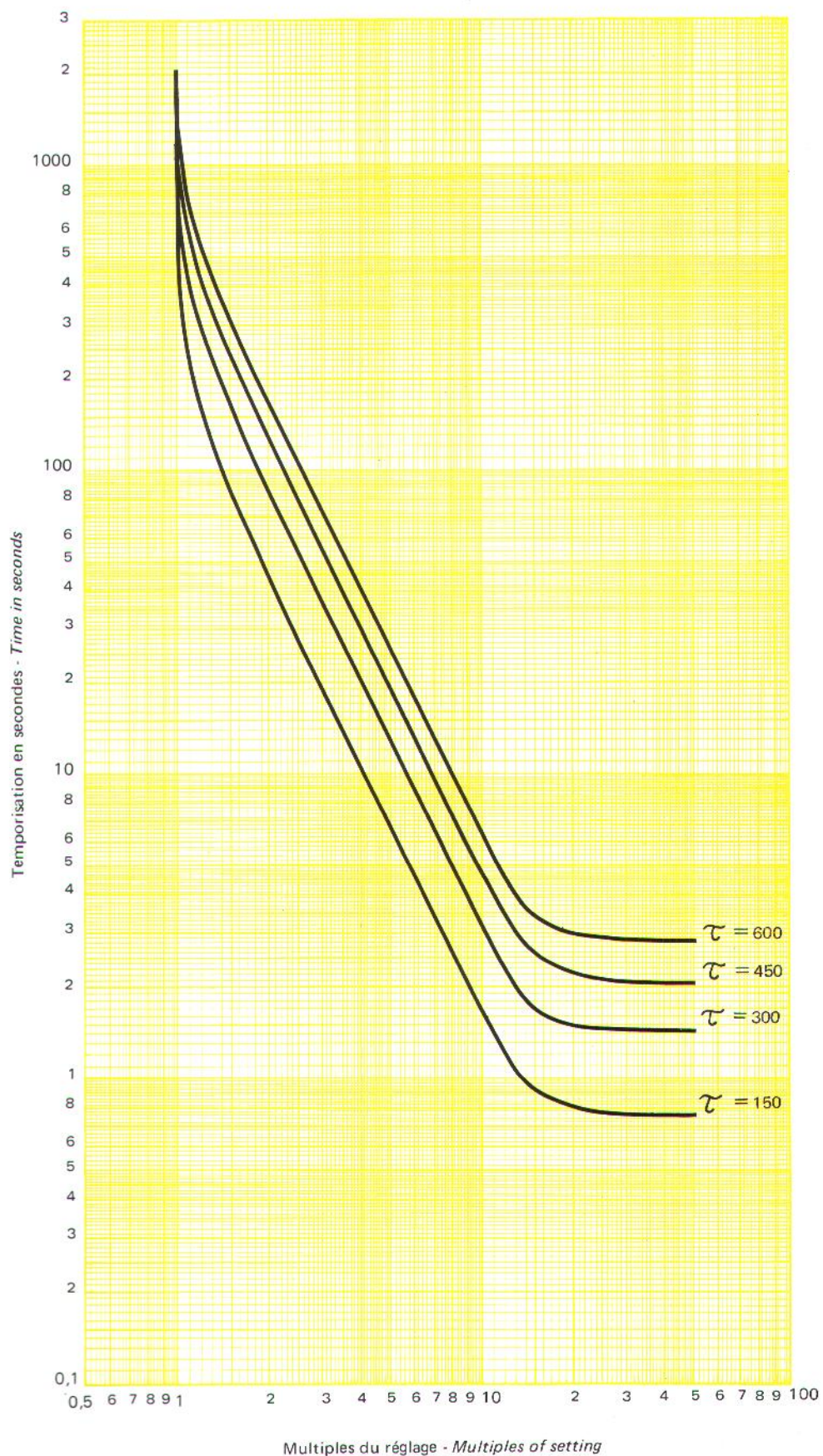
Courbes de fonctionnement Operating curves
