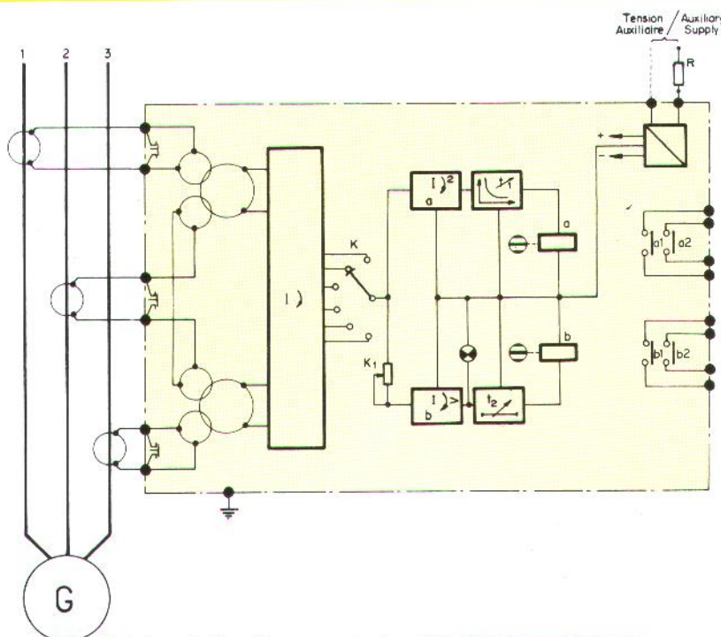
Schéma de fonctionnement simplifié et de raccordement Simplified operation and connection drawing
