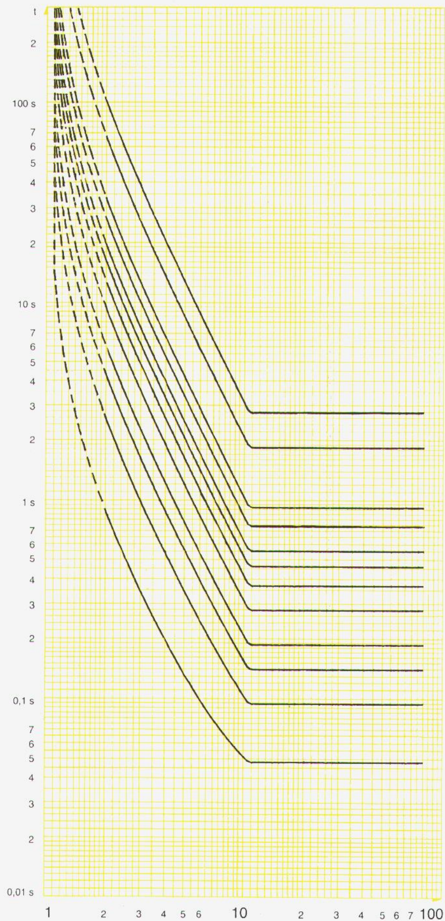
Fig. 4 : ITV 7466 - Courbes à temps extrêmement inverse type C - CEI 255-4 pour 100% U_n ITV 7466 - Extremely inverse time curves to IEC 255-4 type C for 100% U_n .
