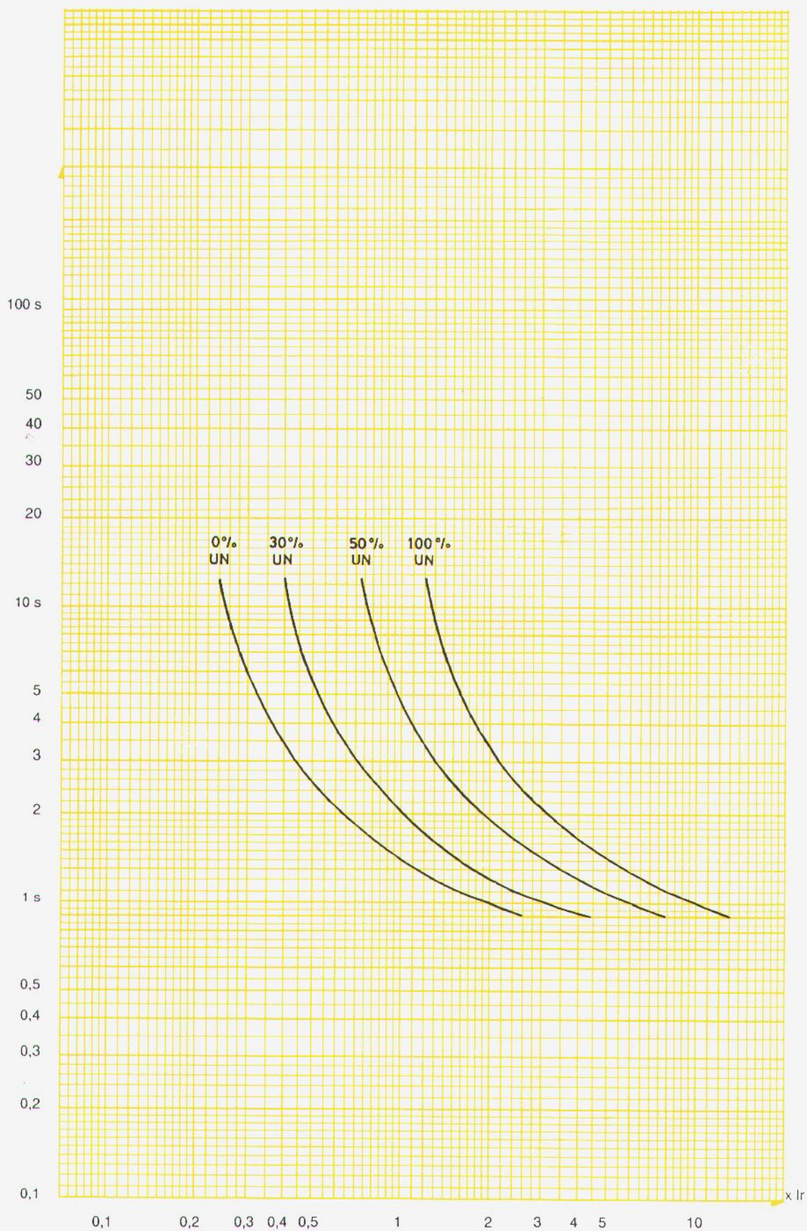
Fig. 6 : ITV 7266 - Exemple de diagramme de fonctionnement pour une courbe t(I >) = 1 s en fonction de la tension ITV 7266 - Example of the operating diagram for a curve t(I >) = 1 s at 10x as a function of the voltage.
