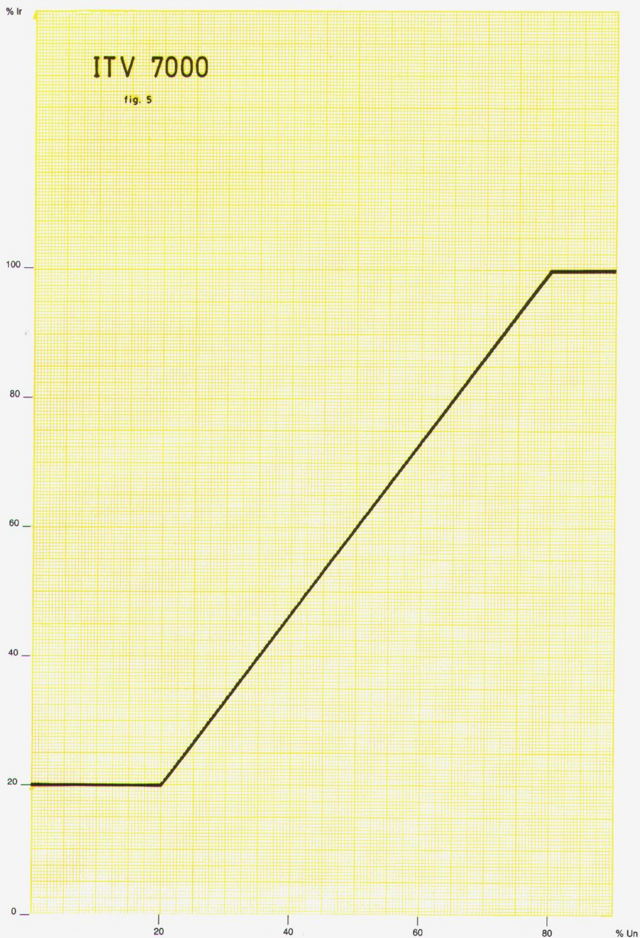
Fig. 5 : ITV 7000 - Evolution des seuils ampéremétriques en fonction de la tension ITV 7000 - Modification of the operating current as a function of the voltage
