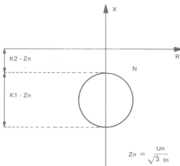
Fig. 1 — YTM 7111 - Diagramme de fonctionnement Operating diagram
